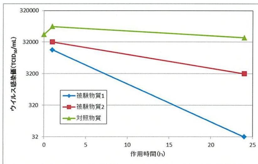
図2 ウイルス不活化試験の結果 (Flu A)
